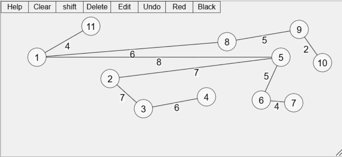
Cây khung nhỏ nhất
